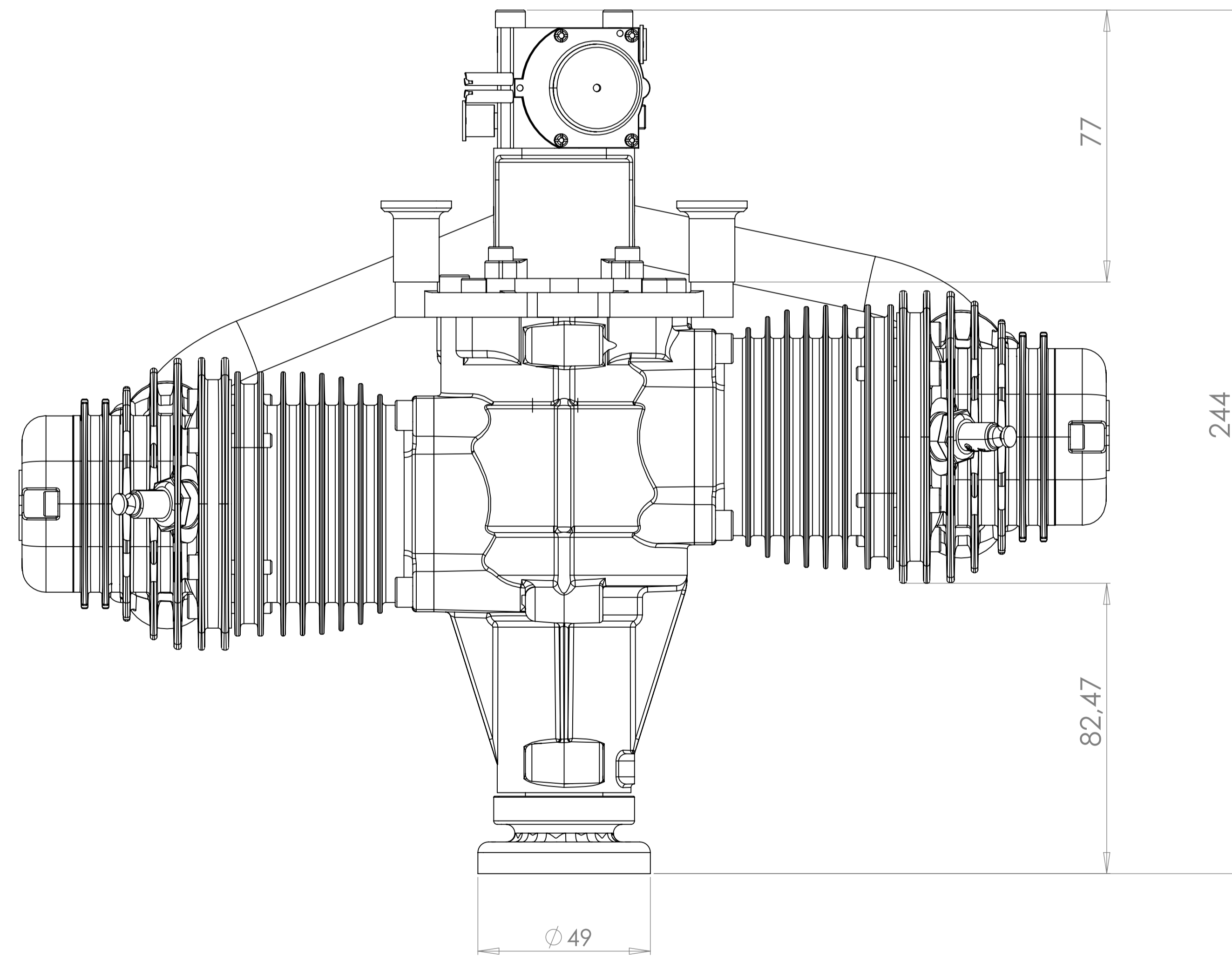
VALACH MOTORS VM 120B2 4T
